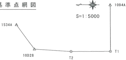
基 準 点 網 図
