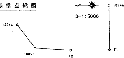
基準点網図
